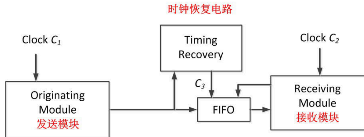
采用FIFO实现近似同步通信
